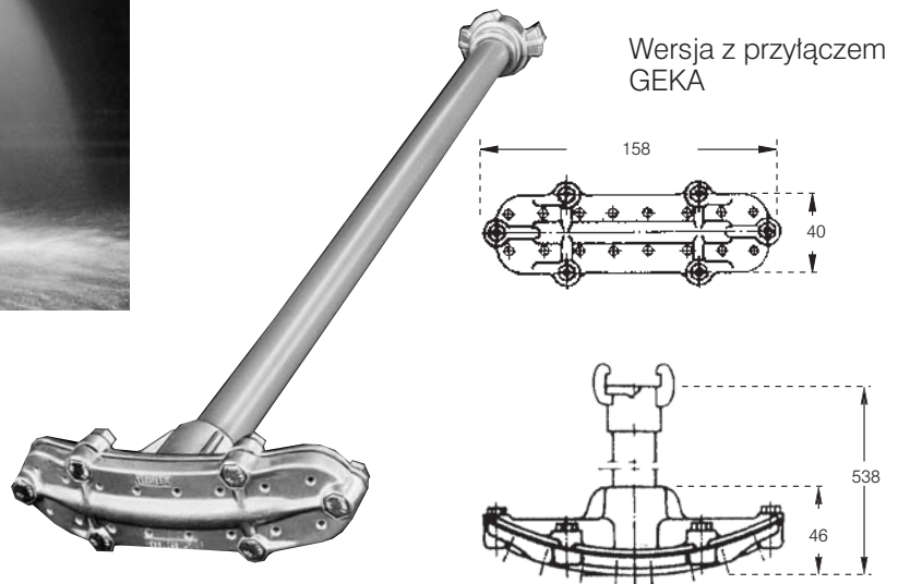
Lanca pistoletowa z przyłączem GEKA Nr kat. 095.016.00.01.76
