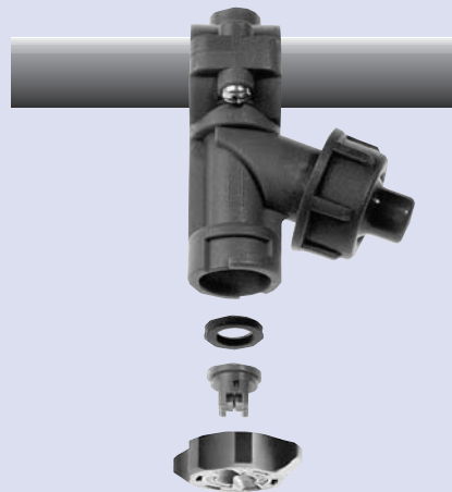
Korpus z membranowym zaworem odcinającym (wersja z obejmą montażową do belek „mokrych“)
