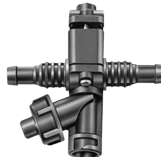
Korpus pojedynczy przelotowy Nr katalog. 275. KL dla rur o \varnothing zewn. 3/4" Nr katalog. 275. KH dla rur o \varnothing zewn. 1/2"
