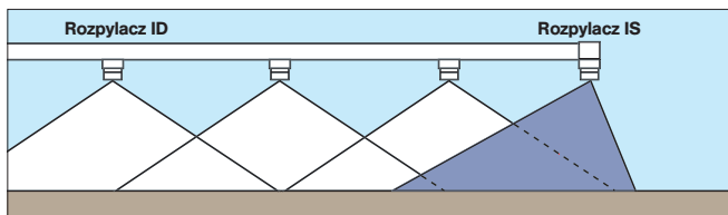
Rozpylacz krańcowy belki
