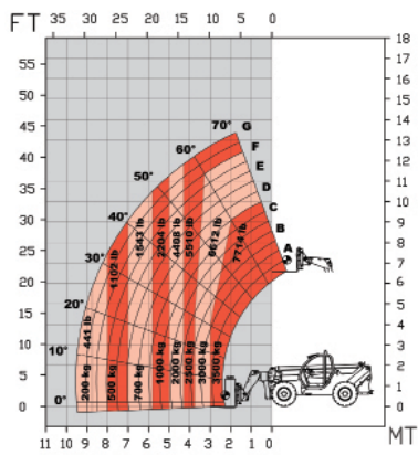
FH 14•42 WHEELS / NA KOŁACH / KEREKEKEN
