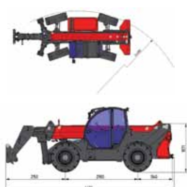
OUTRIGGERS / NA PODPORACH / STABILIZÁTOROKON
