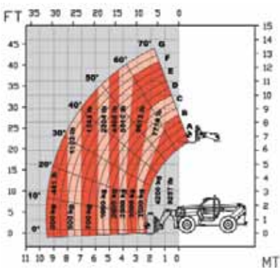
FH 14•42 WHEELS / NA KOŁACH / KEREKEKEN
